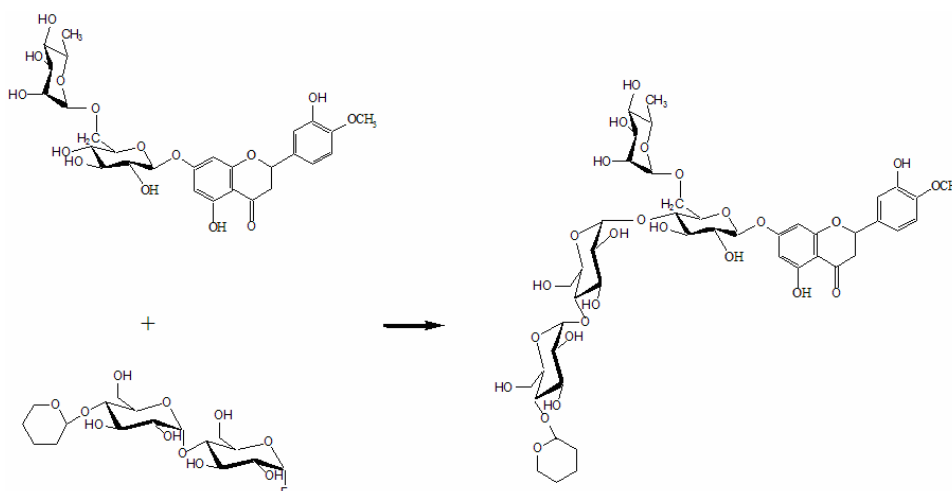
Fig. 3. Réaction de couplage entre l'hésperidine et l' \alpha -fluorure de 4'-tétra-hydropyrano-maltosyle réalisée par l'action catalytique de la CGTase de Bacillus circulans .
