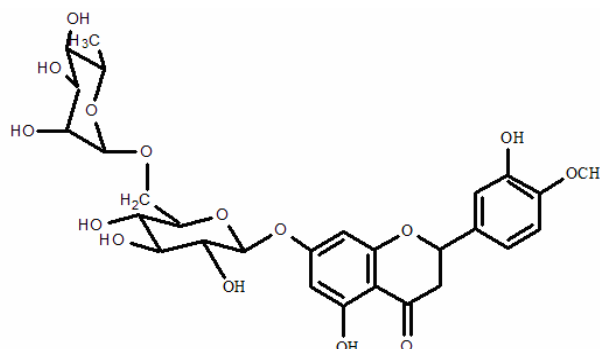
Fig. 2. L'hesperidine.
