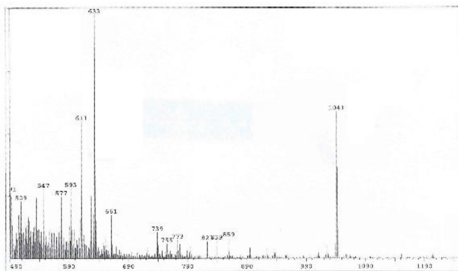
Fig. 6. L'analyse par la spectrométrie de masse de la réaction de transglycosylation de l'hésperidine par l'action catalytique de la CGTase de Bacillus circulans .
