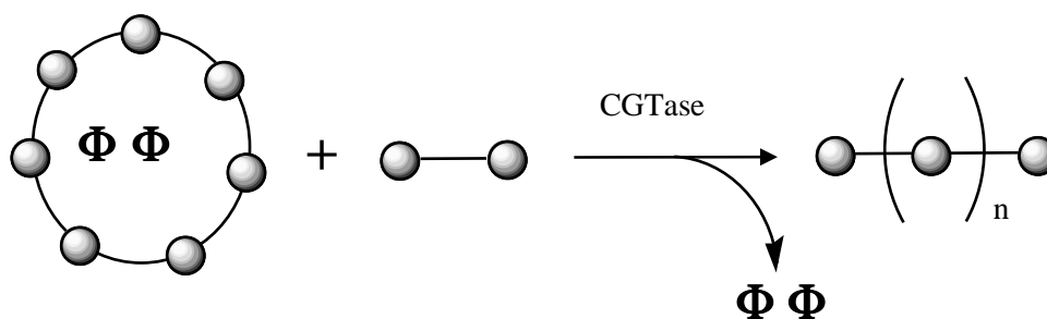
Fig. 4. Réaction de couplage entre la \beta -cyclodextrine et le maltose. \text{O}—\text{O} : \alpha -D-Glcp-(1 \rightarrow 4)-D-Glcp ; \Phi\Phi : phénolphthaléine.
